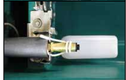
Option I: 1 flotteur MAXIFLOW (l'arrivée d'eau au flotteur est protégée par un câble chauffant 24 V, 20 W, 2 m), 1 résistance 24 V, 180 W
