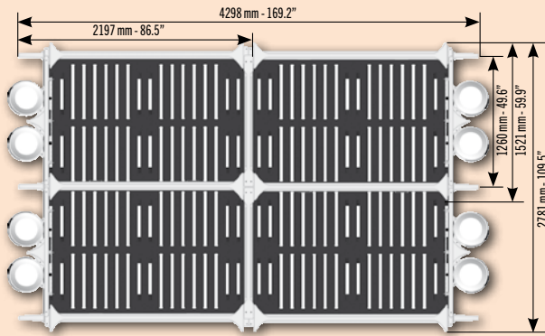
EXEMPLES DE MONTAGE BABY-STAR™ Les cases accolées nécessitent toutes un élément de moins.
